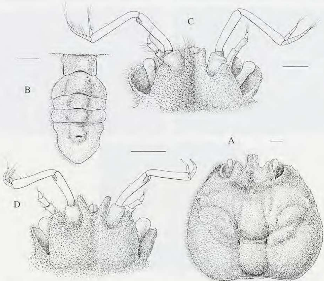
FIG. 3 A-C. — Tymolus daviei sp. nov., ♂ holotype 10 x 11 mm (MNHN-B 25248): A, vue d'ensemble de la carapace; B, face dorsale de l'abdomen; C, bord frontal de la carapace. Échelles = 1 mm.
